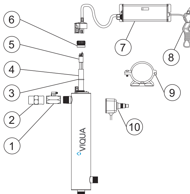
Figure 1 Composants du système
